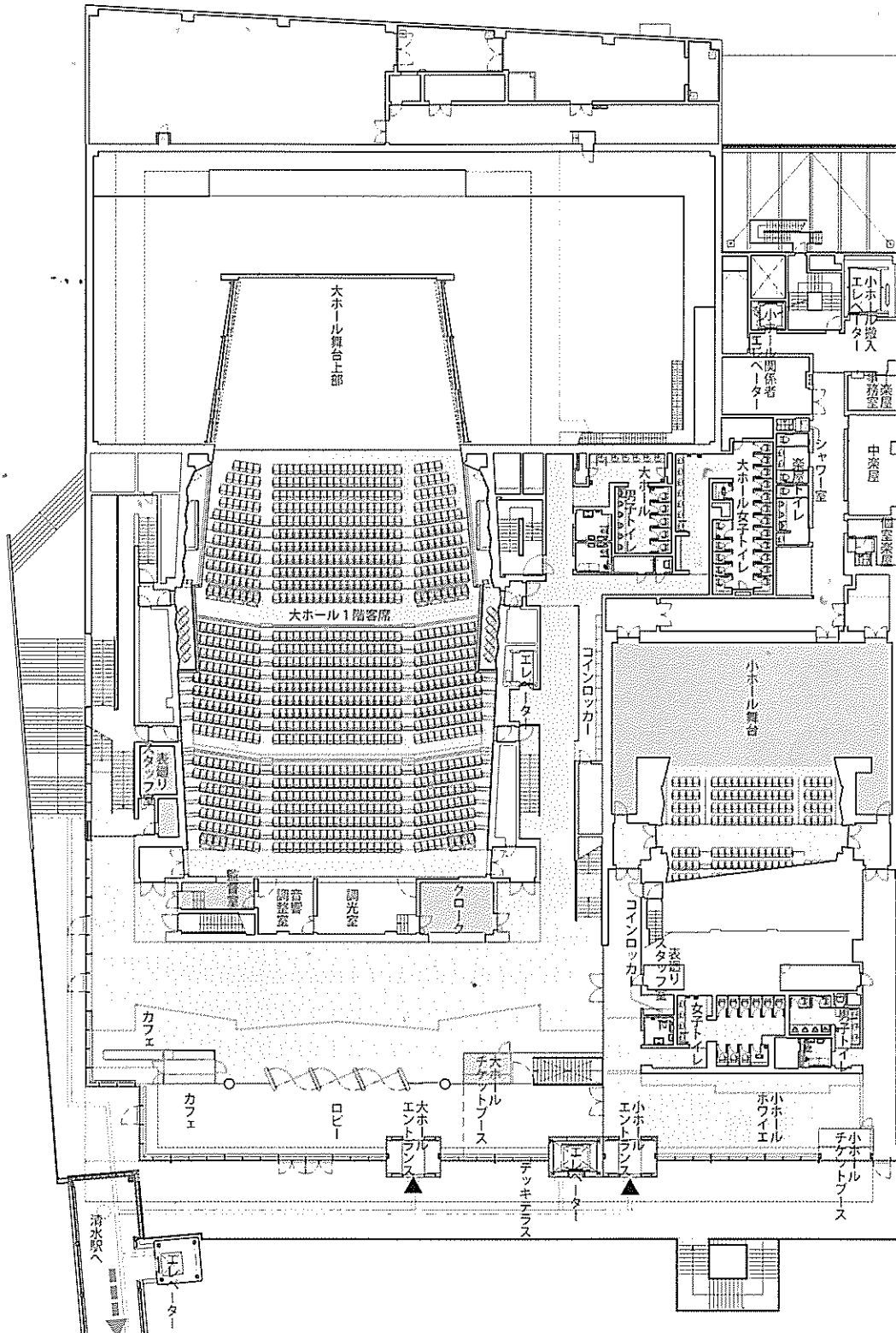
2階平面図
