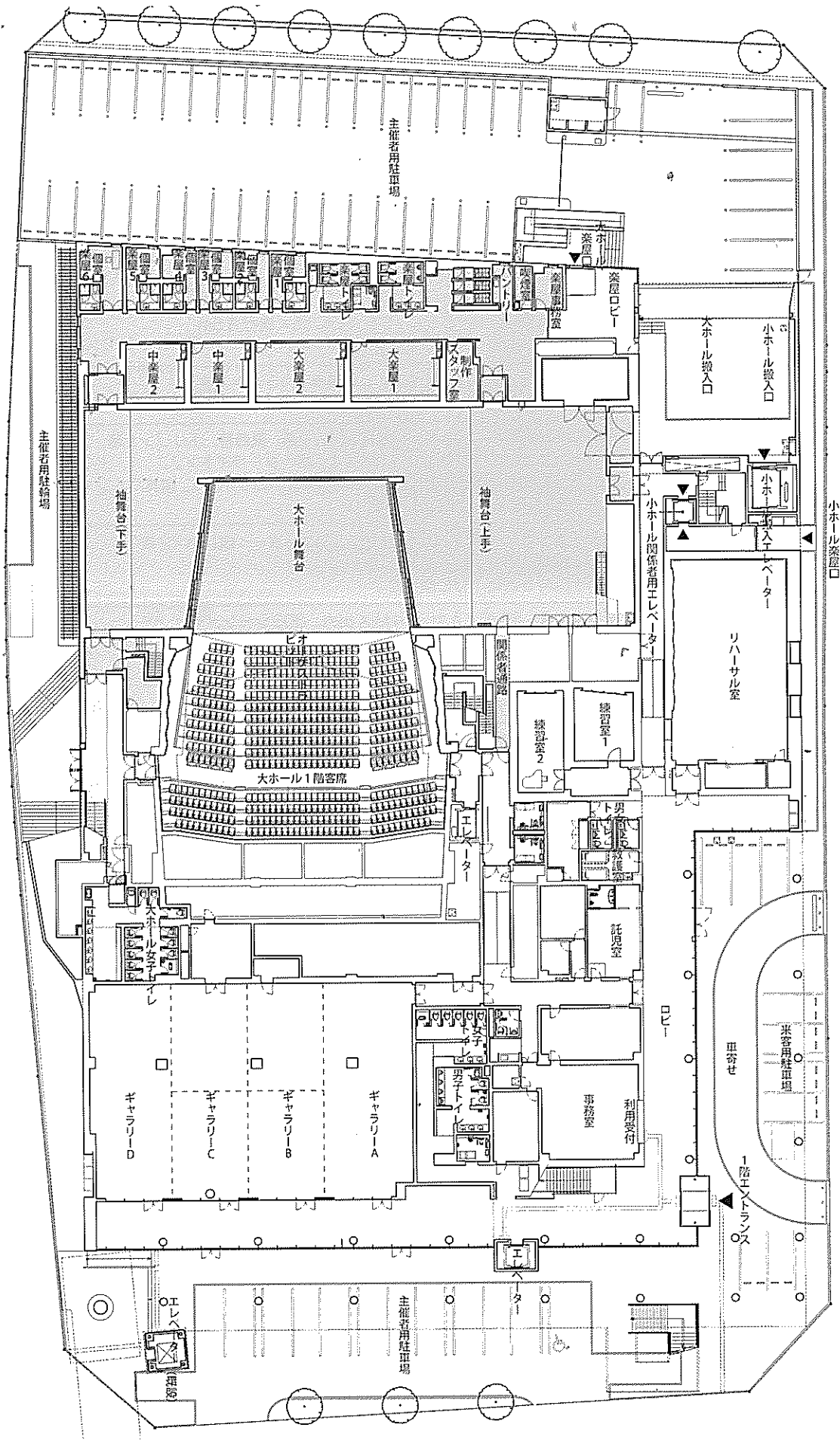
1階平面図
