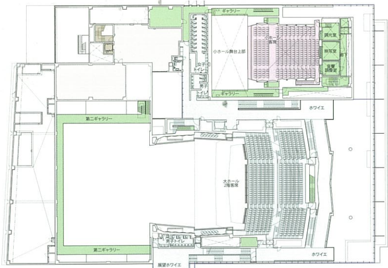
3階平面図
