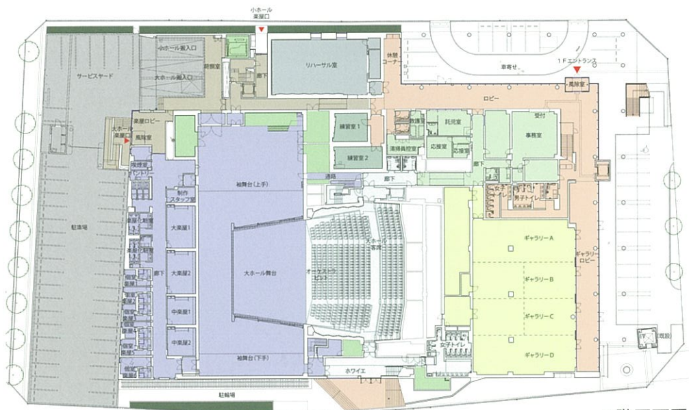
1階平面図
